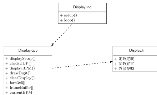
図 17 LEDMatrix のクラス図
